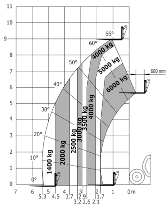
Laaddiagram ruw terrein norm en1459 b Machines op banden met vorken
