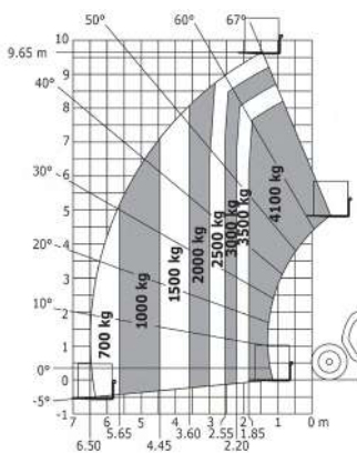
Laaddiagram ruw terrein norm en1459 b Machines op banden met vorken
