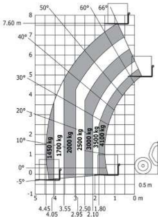
Laaddiagram ruw terrein norm en1459 b Machines op banden met vorken
