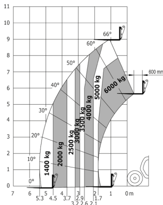
Laaddiagram industrial norm en1459 a Machines op banden met vorken
