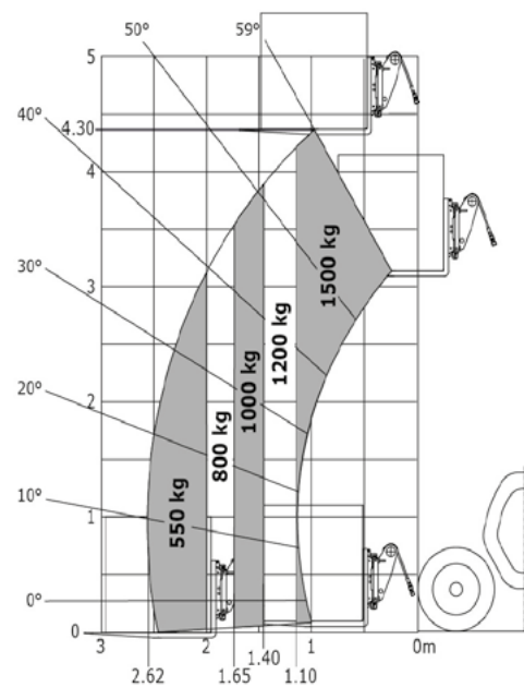
Abaque tout-terrain (EN1459 B) Centre de gravité à 500 mm
